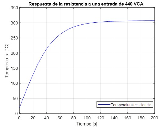
Figura 8. Temperatura de la resistencia a lo largo del tiempo
